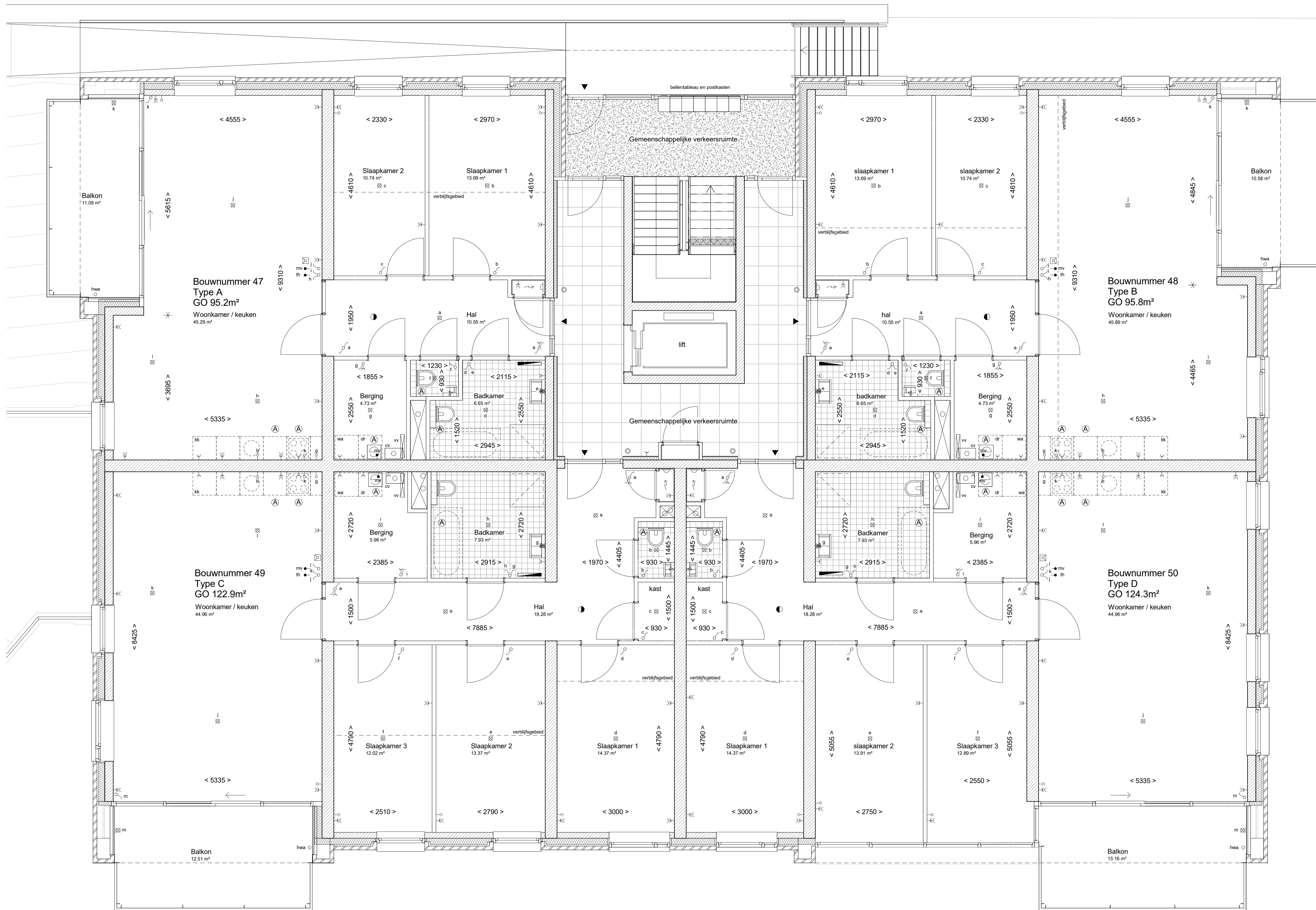
BEGANE GROND schaal 1 : 50
